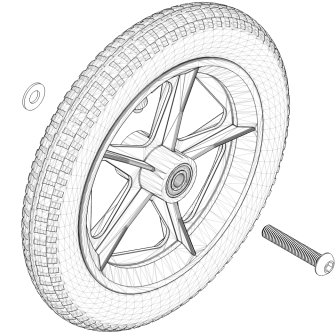
SC-CPLT.007B
