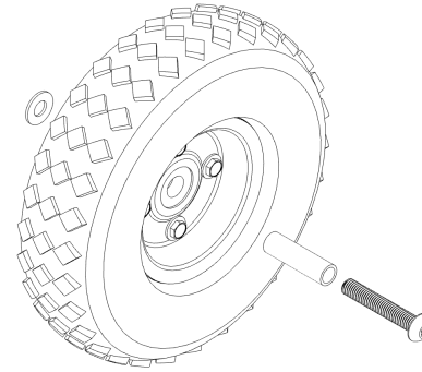
SC-CPLT.007A
