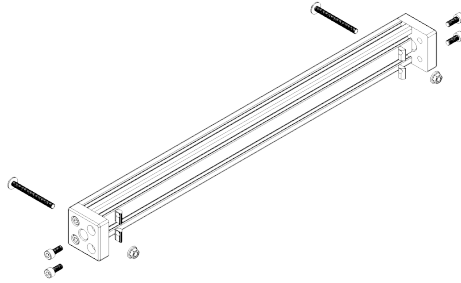
2x SC-CPLT.004
